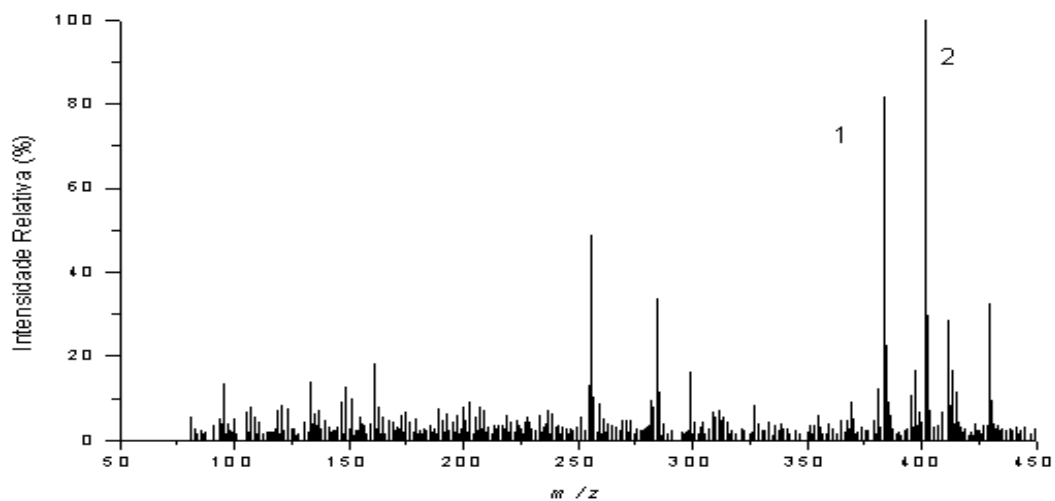
Figura 1b. Cromatograma das amostras de camarão pitu para a detecção de 7-Ceto (Picos 1 e 2).
