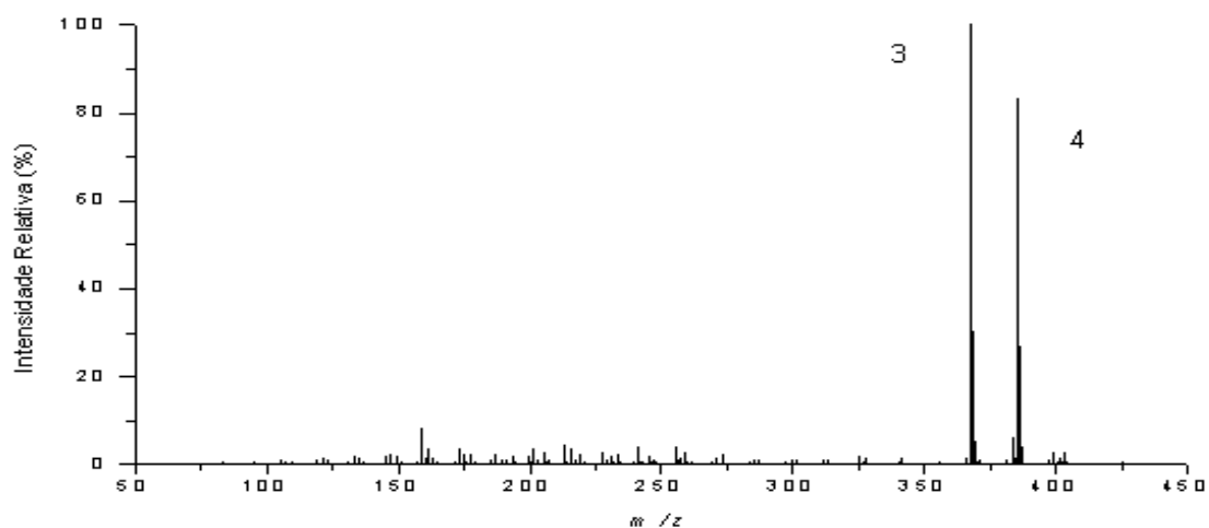
Figura 2a. Cromatograma padrão de Triol (Picos 3 e 4).
