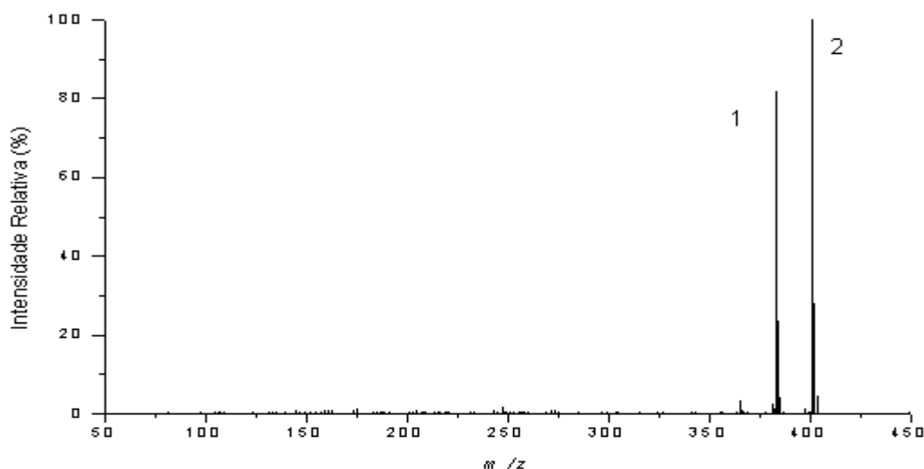
Figura 1a. Cromatograma padrão de 7-Ceto (Picos 1 e 2).
